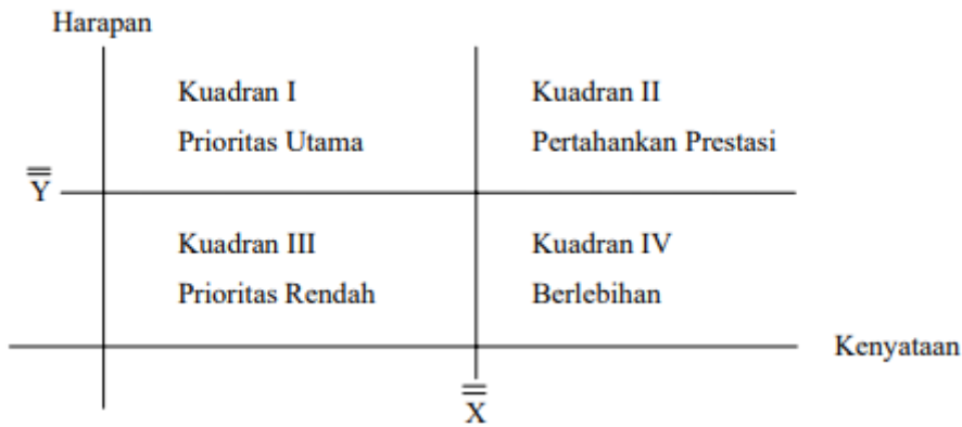
Gambar 3.6. Diagram Kartesius (Supranto, 2001)
