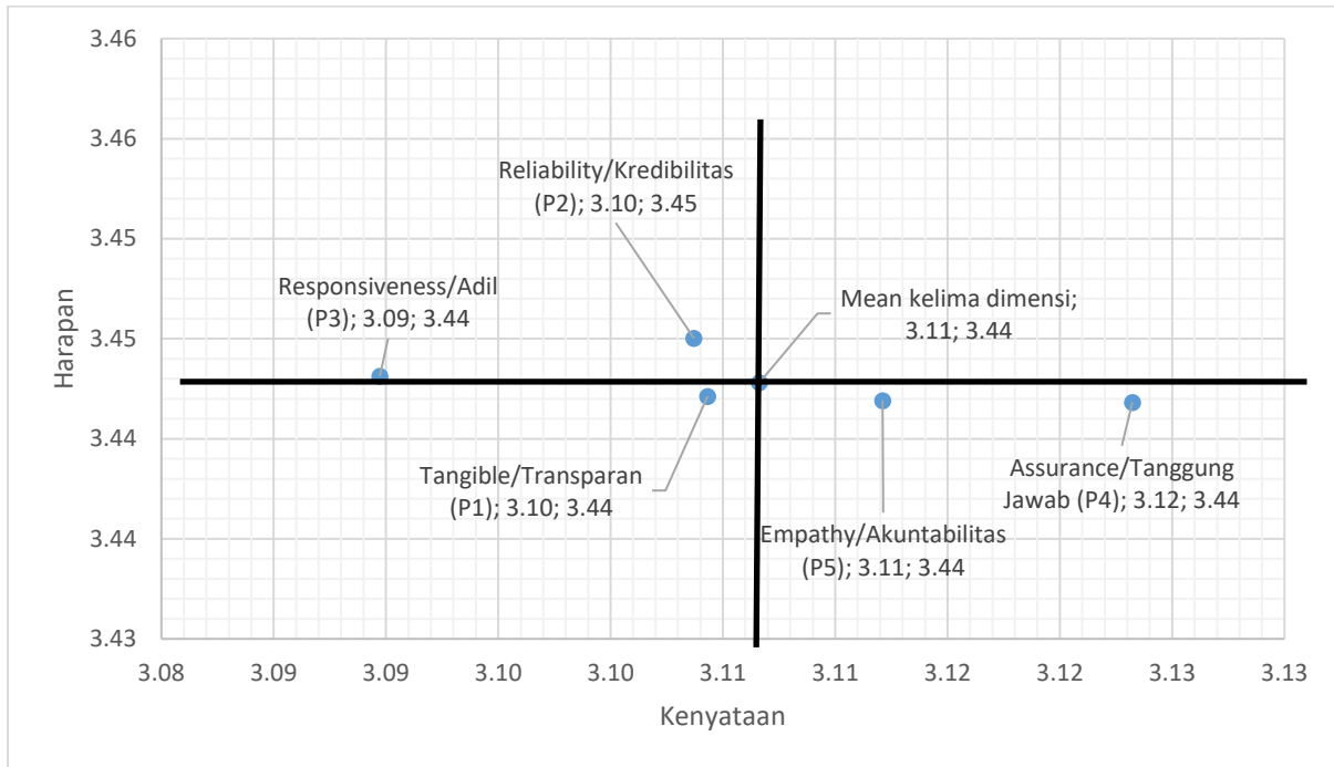
Gambar 3.5. Diagram Kartesius Survei Kualitas Pelayanan kemahasiswaan FBS Unesa Tahun 2020
