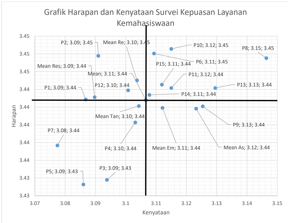
Gambar 3.5. Diagram Kartesius Survei Kualitas Pelayanan kemahasiswaan FBS Unesa Tahun 2020
